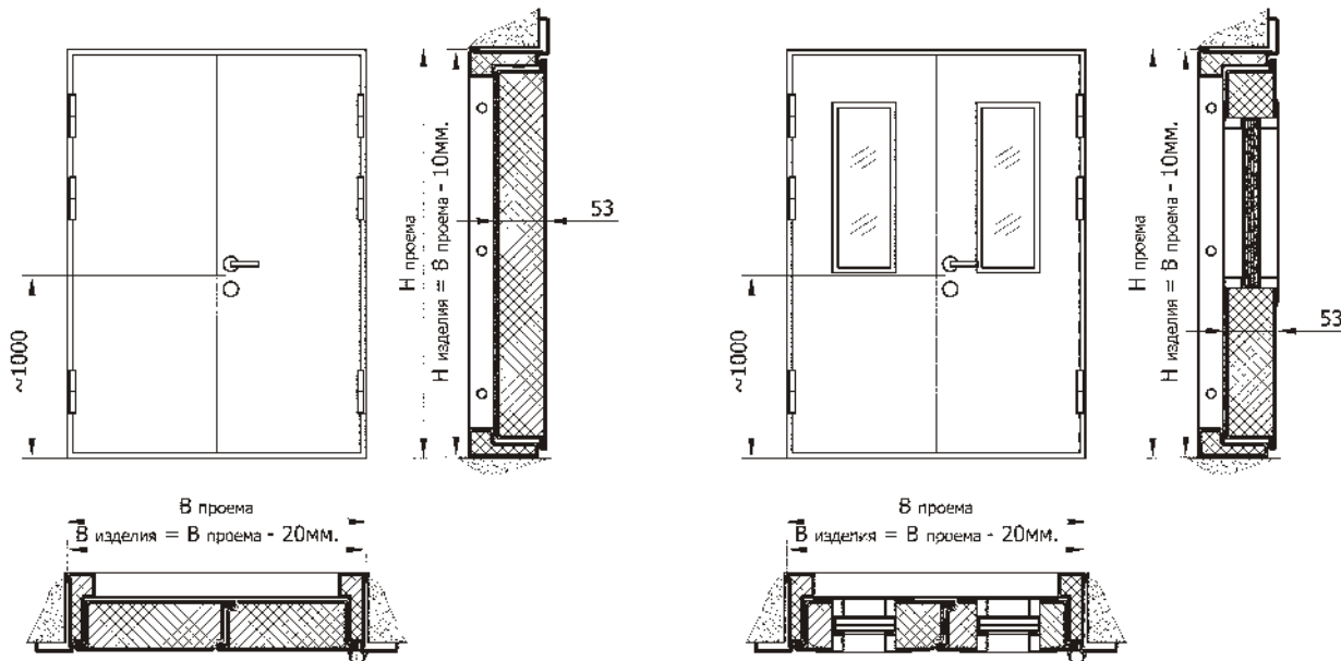
Варианты крепления рамы к проему
