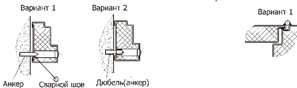
Варианты исполнения полотна .
